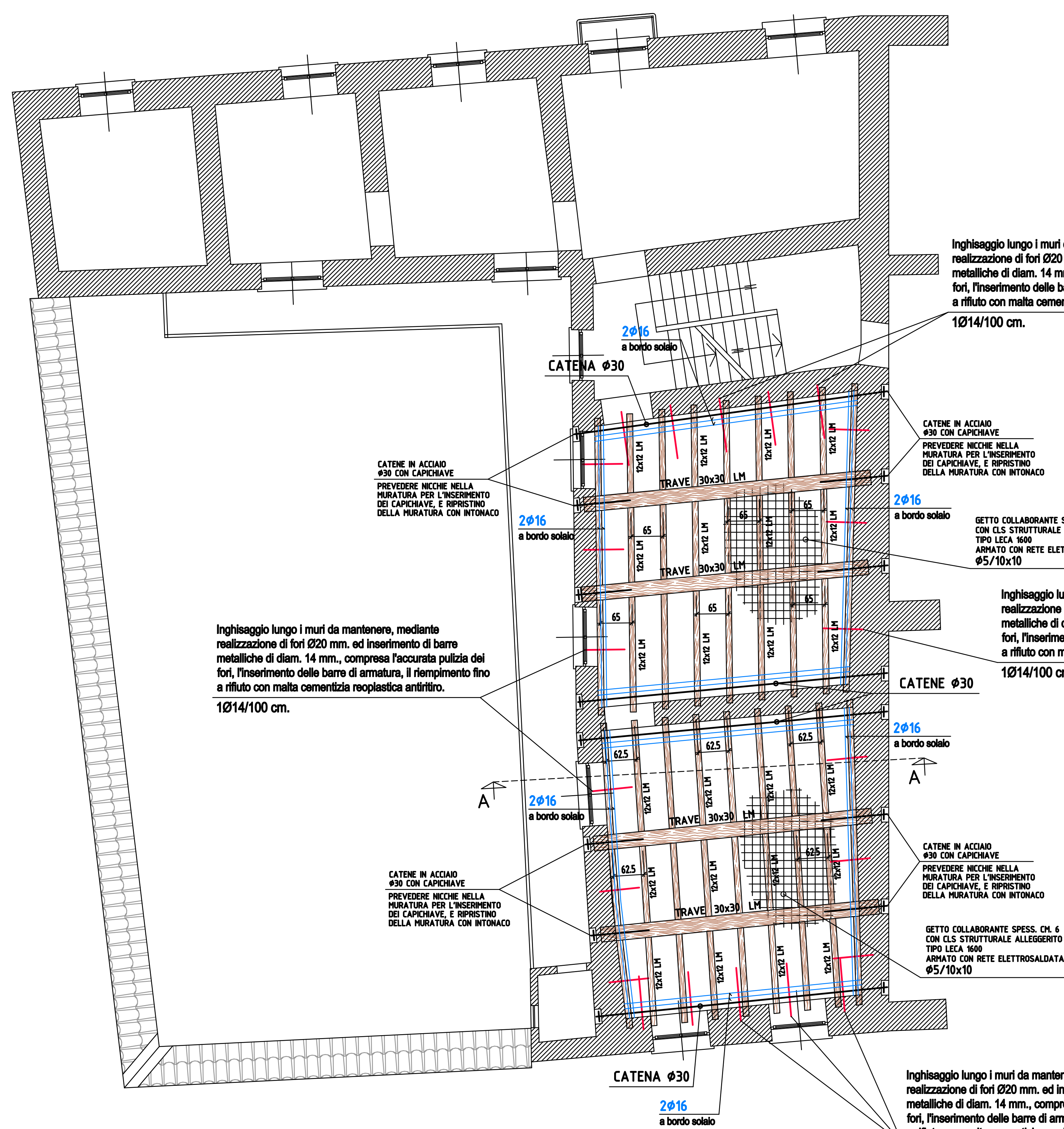
PIANTA SOLAIO PIANO SECONDO IN PROGETTO
