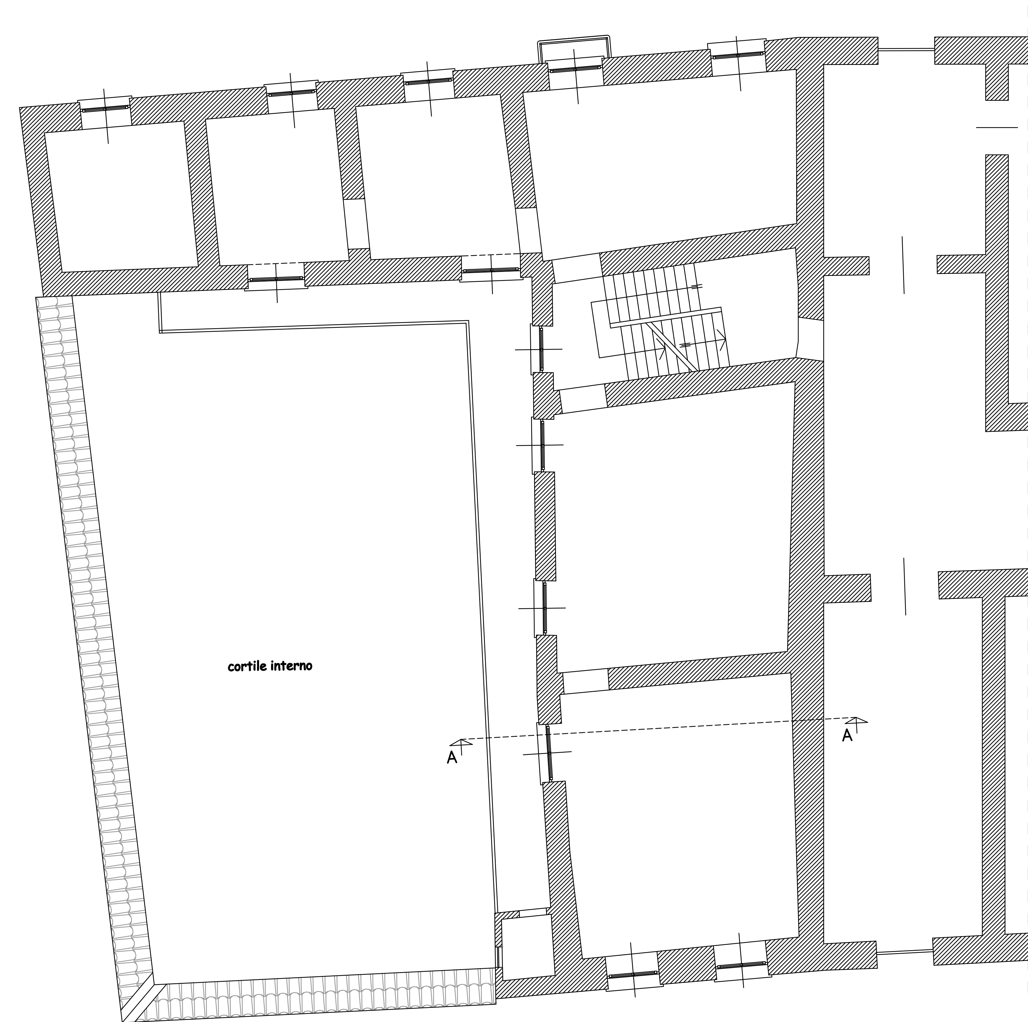
PIANTA MURATURE PIANO PRIMO (INVARIATA) PER APPOGGIO SOLAIO PIANO SECONDO
